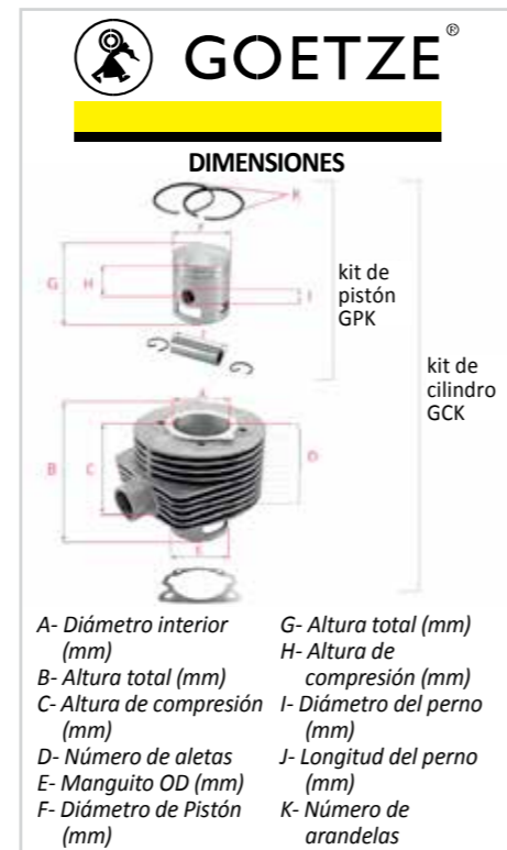
En la imagen, composición de cada kit de componentes de motor Goetze.
